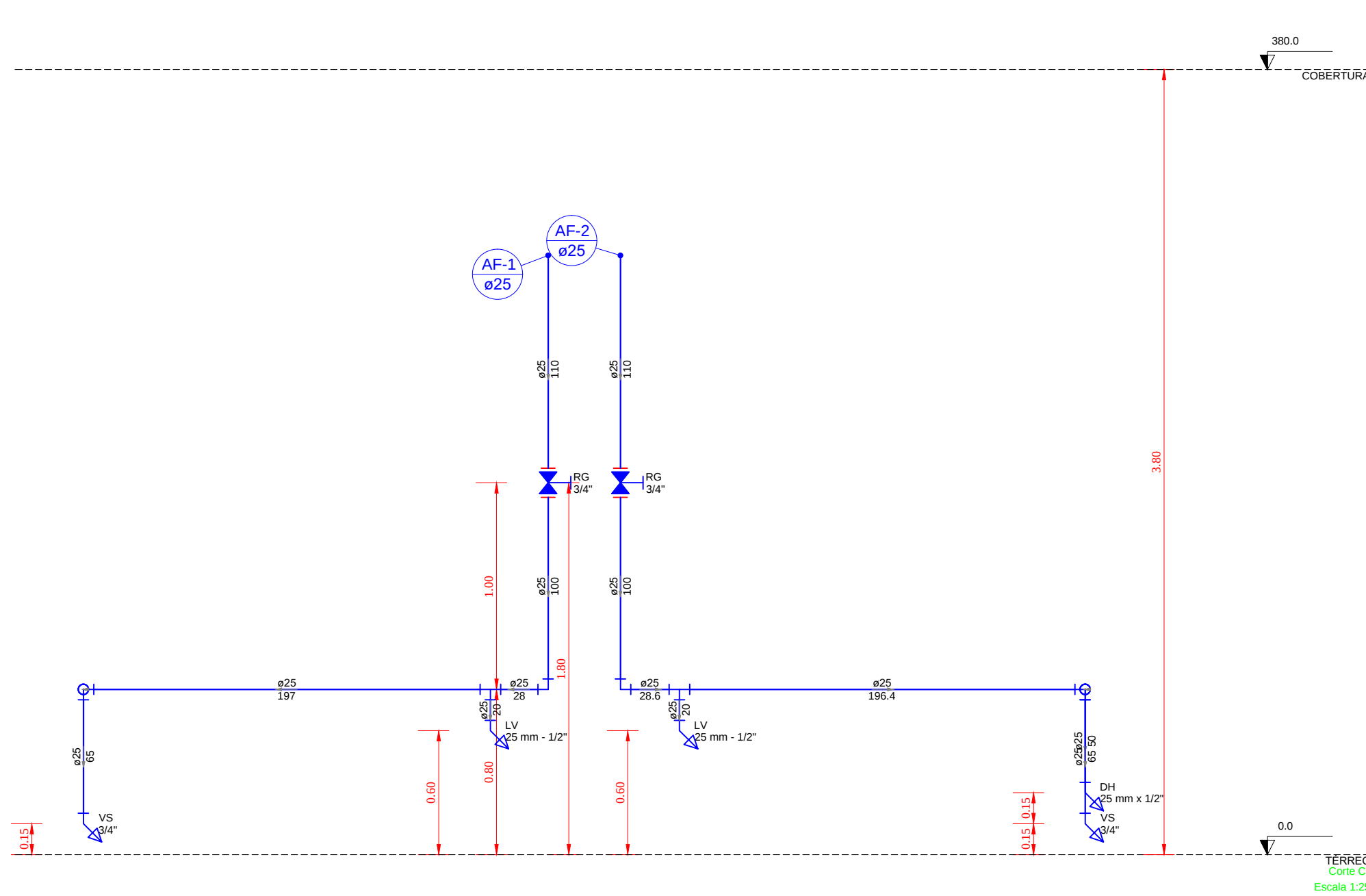
Detalhe H10 Escala 1:25
